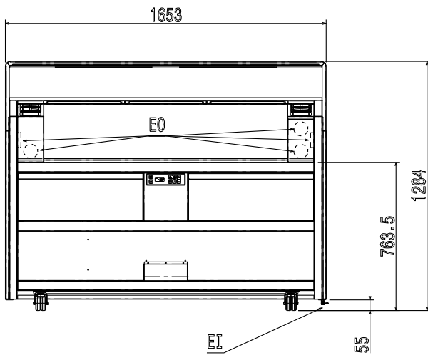
Front aanzicht
